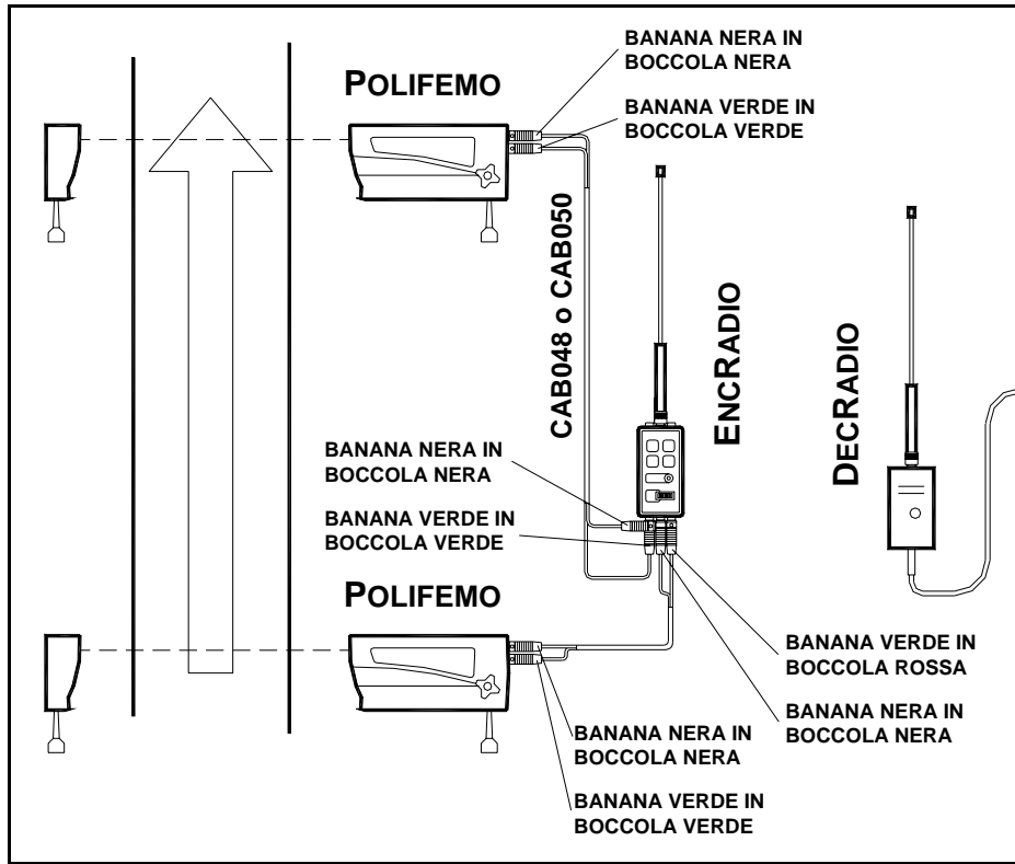
Fig. 18 – Rilevazione velocità
